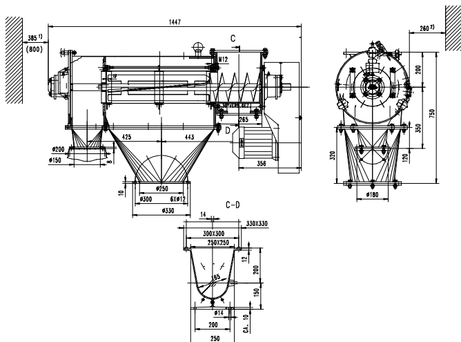
Tamiseur E 650 modèle C1
