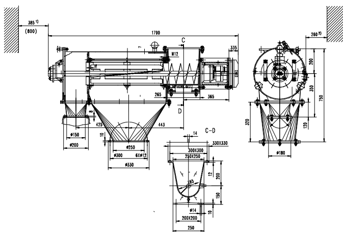
Tamiseur E 650 modèle B1
